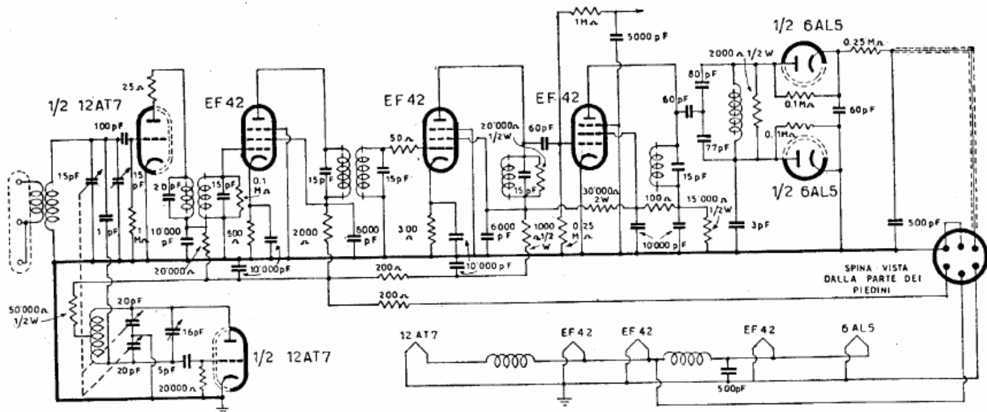
WATT RADIO - Mod. Sintonizzatore FM - 12AT7 oscillatrice e miscelatrice. Prime due EF42 amplif. MF a 10,7 Mc. Terza EF42 limitatrice. Rivelatore e discriminatore con 6AL5. Gamma 88-108 Mc. Collegabile al mod. Giubileo FM.
